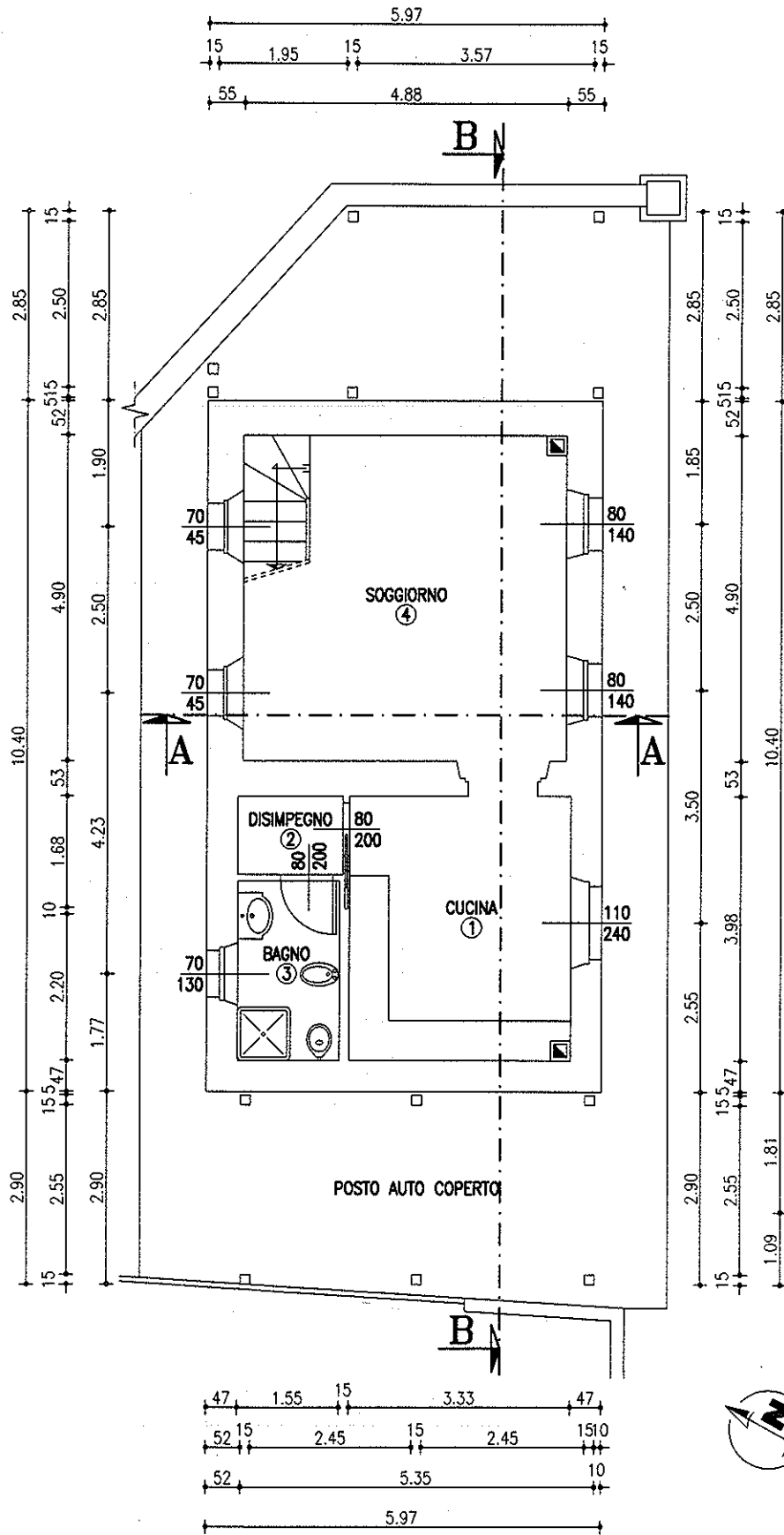
DATI PARAMETRICI DEI VANI - PIANO TERRA -
