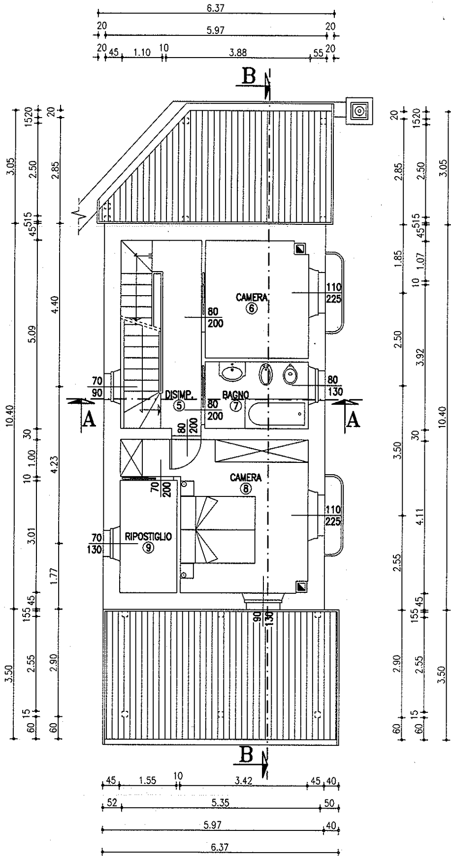
DATI PARAMETRICI DEI VANI - PIANO PRIMO -
